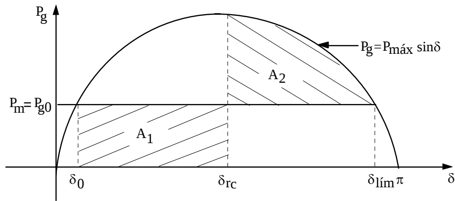
Figura 6.21.- Determinación del ángulo crítico de aclaramiento
