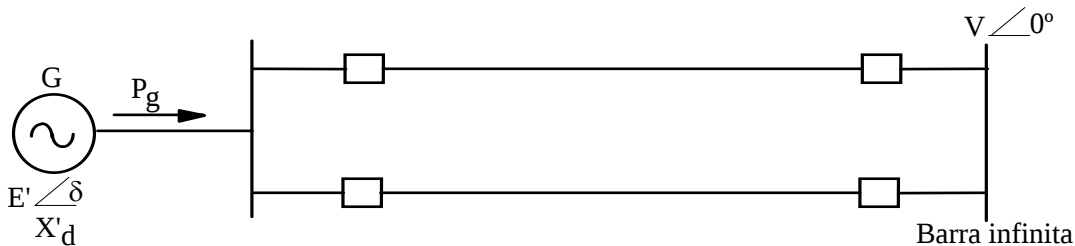
Figura 6.1.- Sistema generador-línea-barra infinita
