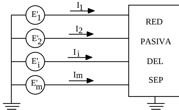
Figura 6.6.- Sistema multigenerador
