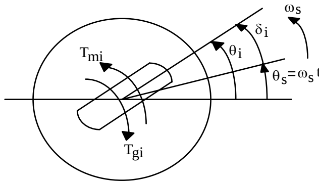
Figura 6.5.- Representación esquemática de un generador síncrono
