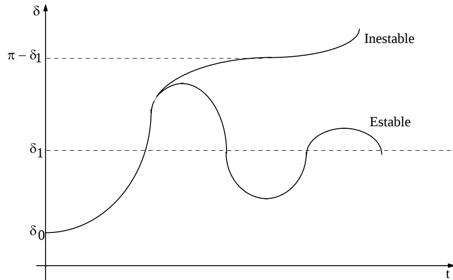
Figura 6.3.- Curvas de oscilación de una máquina síncrona
